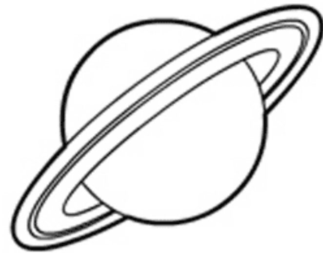
Saturno
